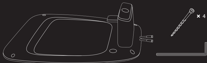
station de chargement et kit d'installation
